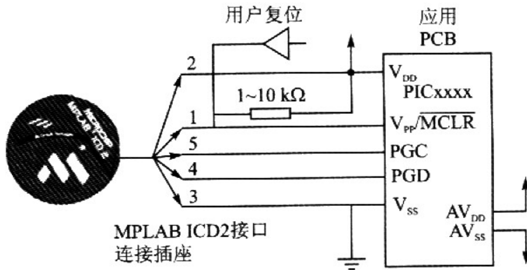
图 1 MPLAB ICD2 与目标板的连接
