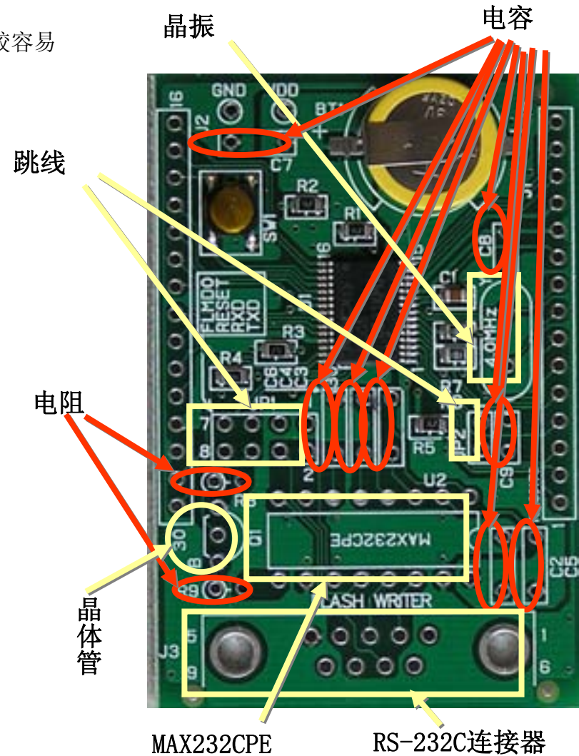
零部件的安装位置如上图所示
