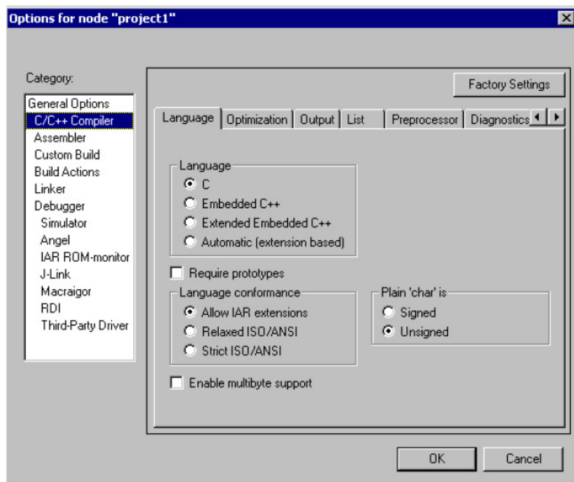
图 5. C/C++ Compiler 选项窗口
