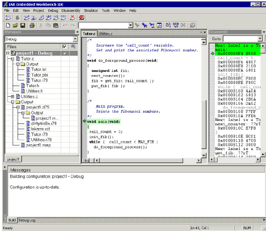
图 11. C-SPY 调试窗口
